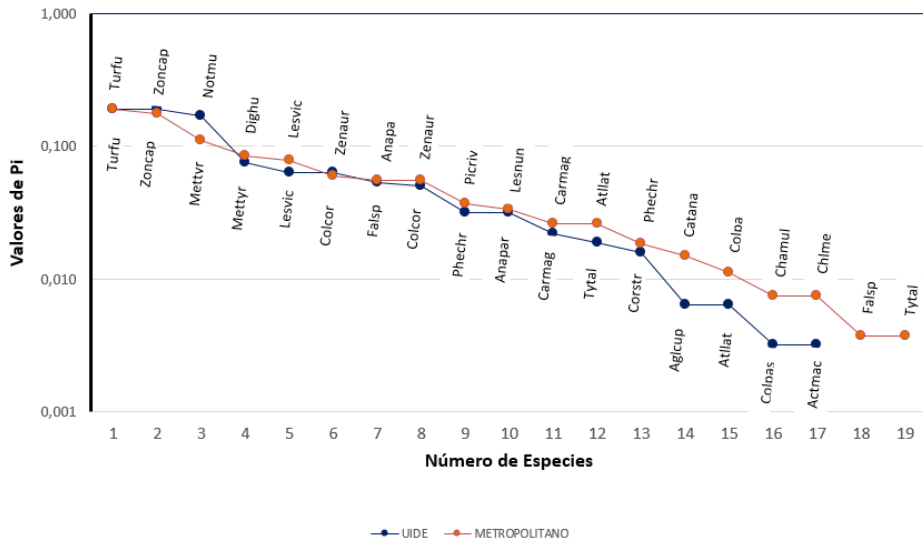
Figura 9.- Curvas de abundancia-diversidad para las dos zonas de estudios (UIDE y Parque Metropolitano Guanguiltagua). Acrónimos: Turfu= Turdus fuscater ; Zoncap= Zonotrichia capensis ; Notmu= Notiochelidon murina ; Mettyr= Metallura tyriantithina ; Lesvic= Lesbia victoriae ; Zenaur= Zenaida auriculata ; Falspa= Falco sparverius ; Colcor= Colibri coruscans ; Phechr= Pheucticus chrysogaster .
