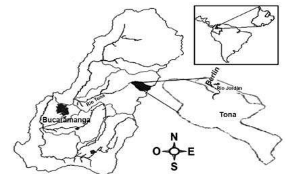
Figura 1. Sitio de estudio en el río Jordán, corregimiento de Berlín, municipio de Tona (Santander), Colombia (modificado de Mendoza y Orozco 2005, Osorio y Salazar 2006)
