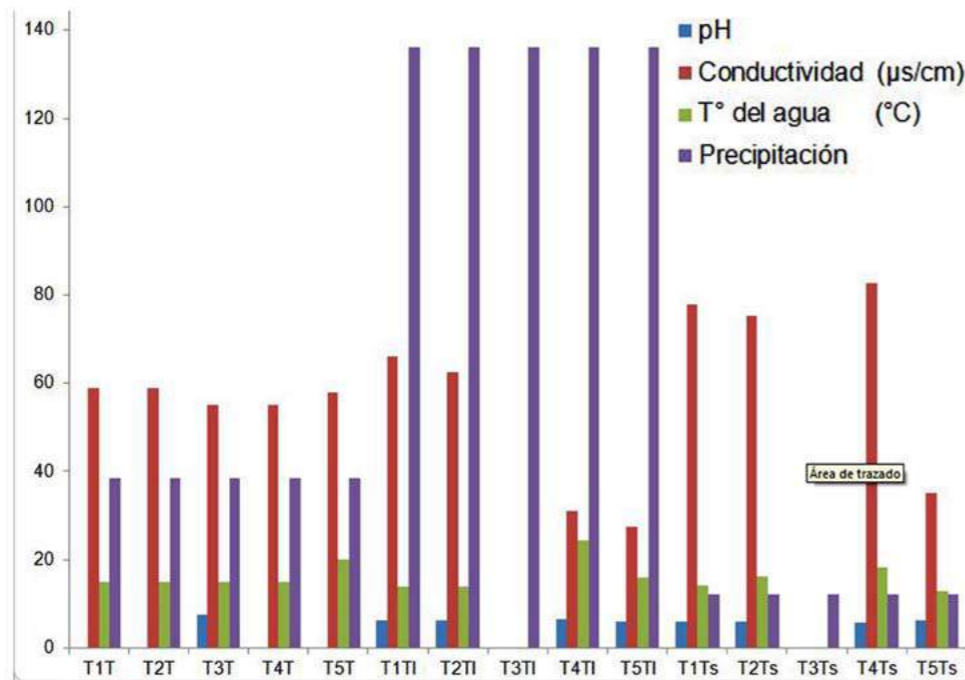
Figura 5. Valores puntuales de pH, conductividad, temperatura del agua [ T^{\circ} , ( ^{\circ}\text{C} )] y precipitación en las temporadas de transición, lluvias y sequía en las diferentes zonas de la represa de Berlín (Santander), Colombia
